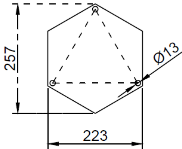
Схема основания светильника
