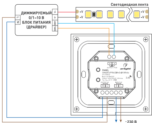
Рисунок 2. Схема подключения панели SMART-P98-DIM-G-IN с использованием выхода «AC OUT»
