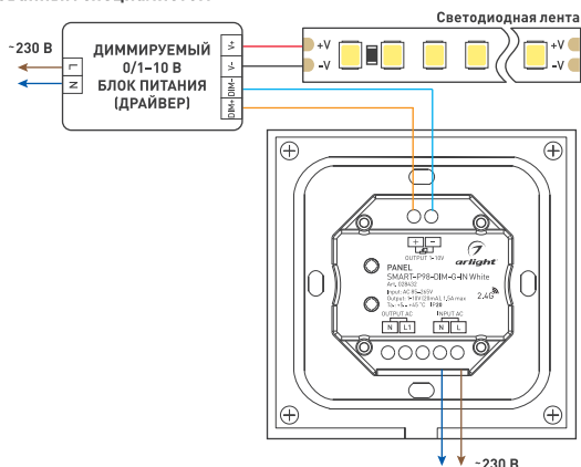
Рисунок 1. Схема подключения панели SMART-P98-DIM-G-IN без использования выхода «AC OUT»
