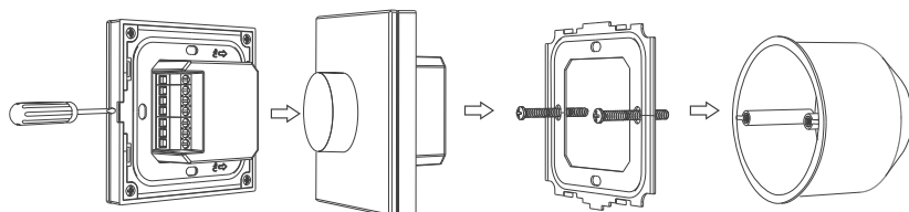
Рисунок 3. Монтаж панели
